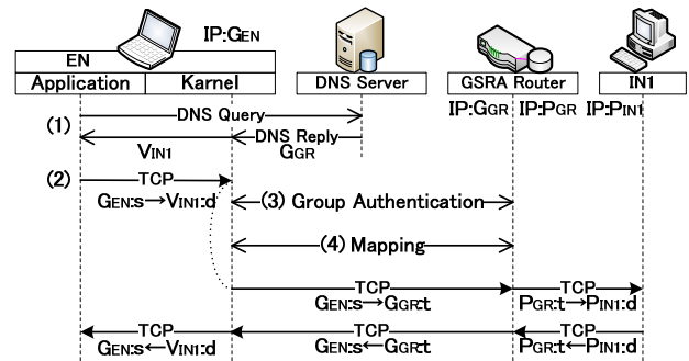
図 2 通信シーケンス
