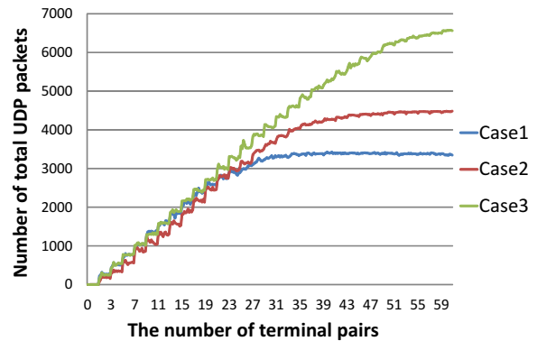
図 8 UDP 通信パケット数の推移
