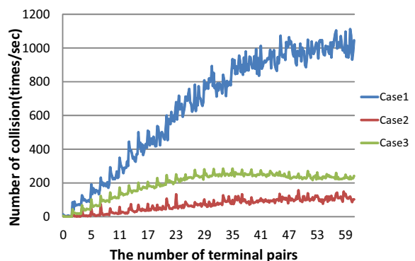
図 9 背景負荷量に対する衝突回数の推移
